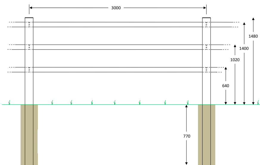
Poda Texas omheining met 3 liggers Leverbaar in verschillende hoogtes.
