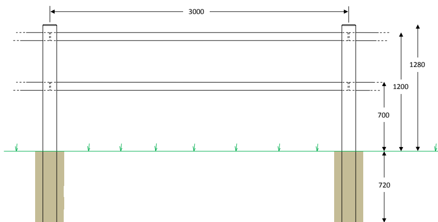
Poda Texas omheining met 2 liggers Leverbaar in verschillende hoogtes.
