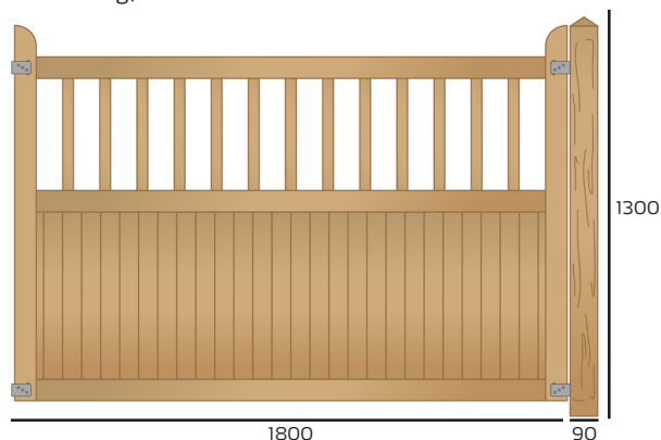
Omheining, achterkant
