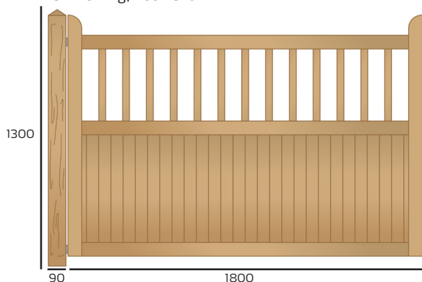
Omheining, voorkant
