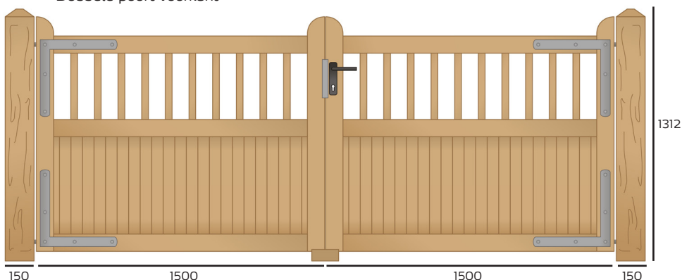
Dubbele poort voorkant
