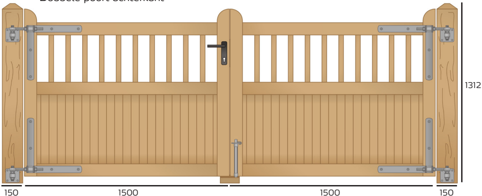
Dubbele poort achterkant
